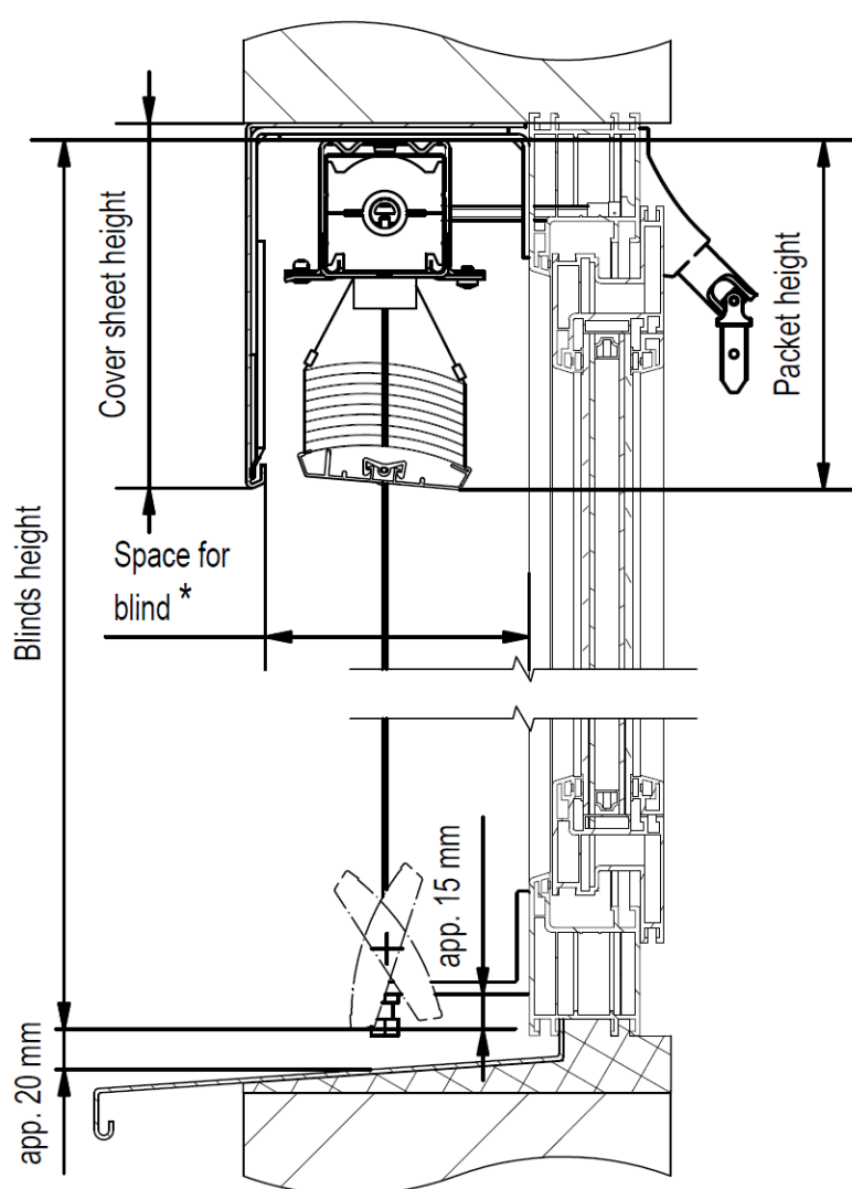
Blind cross section - Τομή περσίδας
