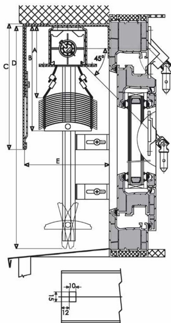
Blind cross section - Τομή περσίδας
