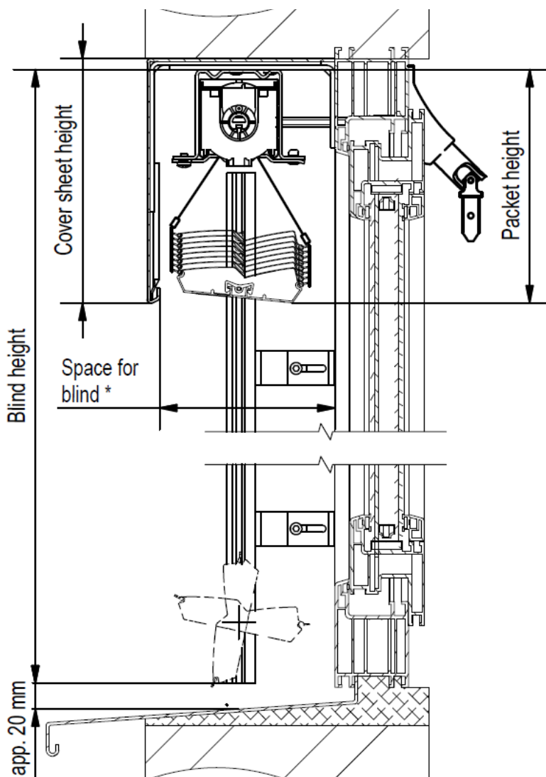
Blind cross section - Τομή περσίδας
