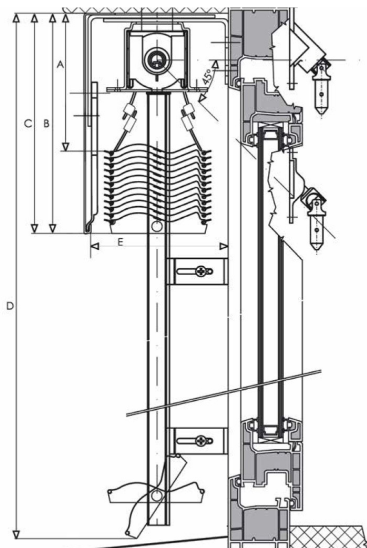
Blind cross section - Τομή περσίδας
