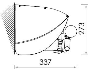
Montaggio con tettuccio Installation with a hood
