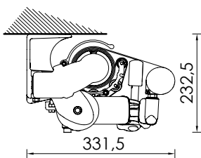
Montaggio a soffitto Ceiling installation
