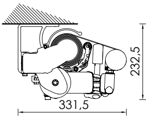
Montaggio a soffitto con staffa estrusa Ceiling installation with extruded bracket
